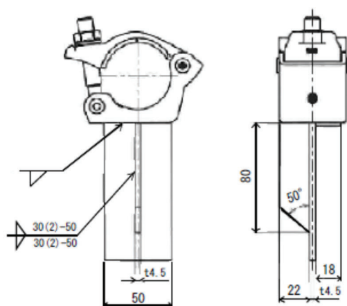
■ 正面図・右側面図 (カバーを外した状態)
